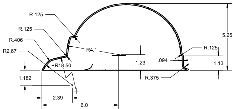
SECTION A-A SCALE 1 : 3
